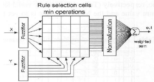
شکل ۲. ساختار سیستم فازی TSK [۴۲]
